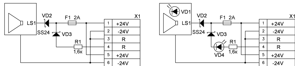
а) BC-07e-Ex-3-24VDC
