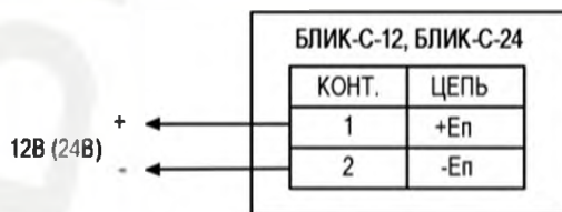
Рис. 1. Схема подключения.
